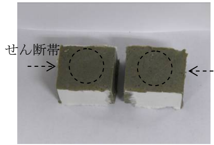
写真-9 せん断帯を含む 供試体
