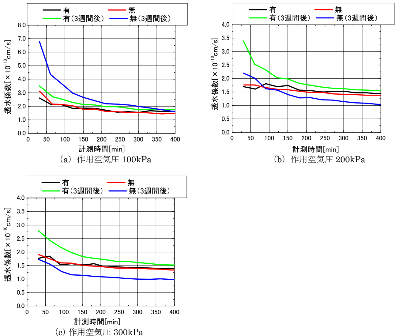
図-9 せん断後の経過時間による比較
