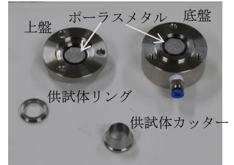
写真-7 小型モールドの解体
