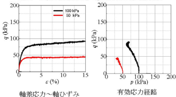
図4 不攪乱縦方向 B3 - ⑤試料の三軸試験結果
