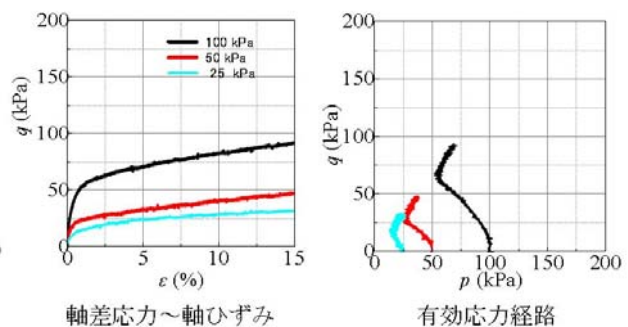
図3 不攪乱横方向 B3 - ④試料の三軸試験結果
