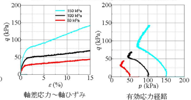
図5 不攪乱横方向 B3 - ⑤試料の三軸試験結果
