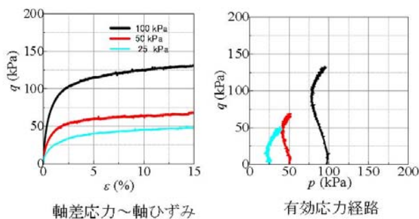
図2 不攪乱縦方向 B3 - ④試料の三軸試験結果
