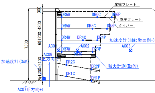
図 1 補強土壁内の計測機器の設置状況
