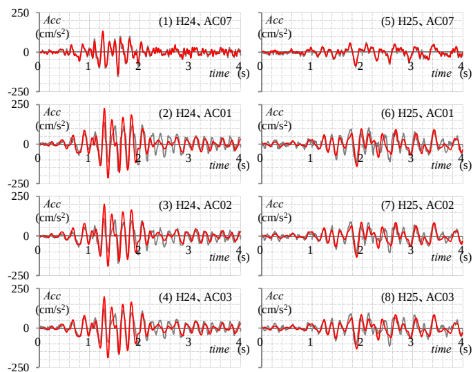
図3 計測加速度の時刻歴 (赤：解析、黒：計測)
