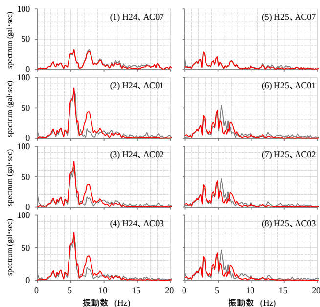
図4 フーリエ解析結果 (赤：解析、黒：計測)
