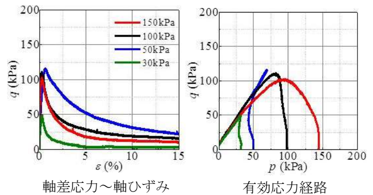
図3 S川 CU試験結果
