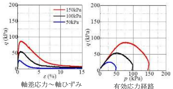
図5 M川 CU試験結果
