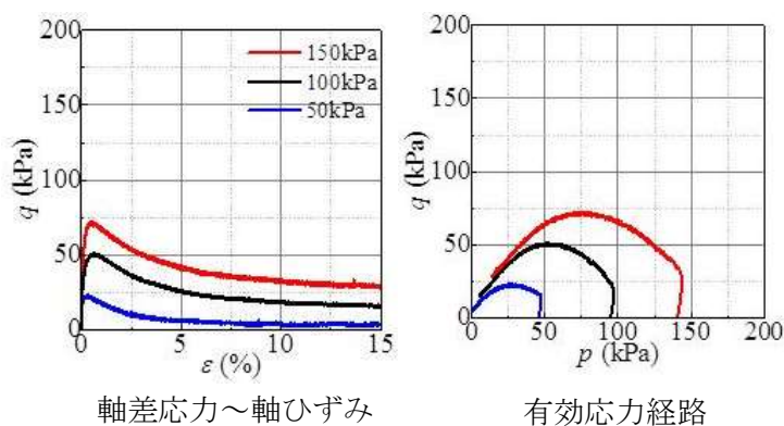
図2 O川 CU試験結果
