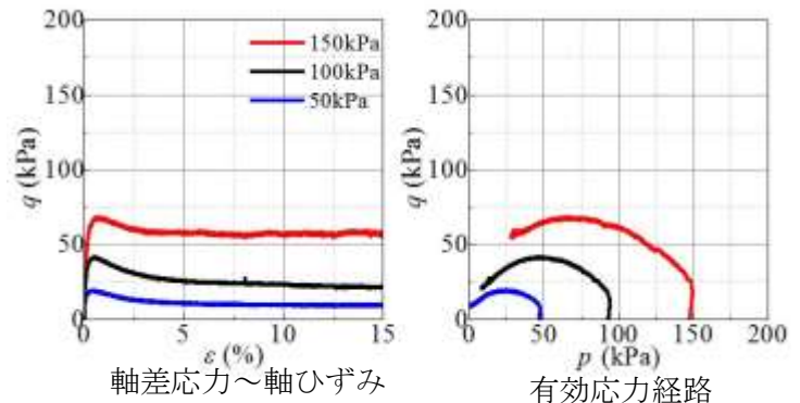
図4 M川 CU試験結果
