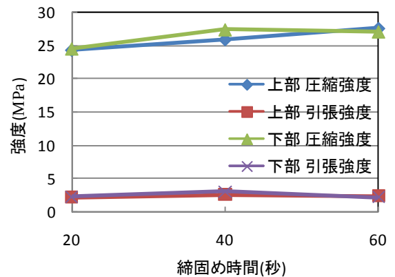
図-5 ラス型枠スランプ 8cm による場合
