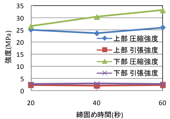
図-4 合板型枠スランプ 18cm による場合
