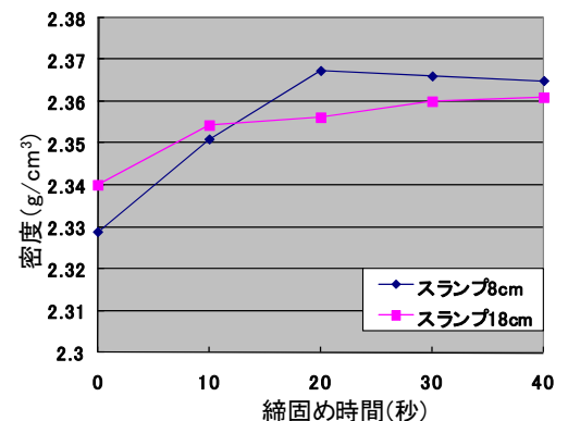
図-2 締固め時間の変化による密度
