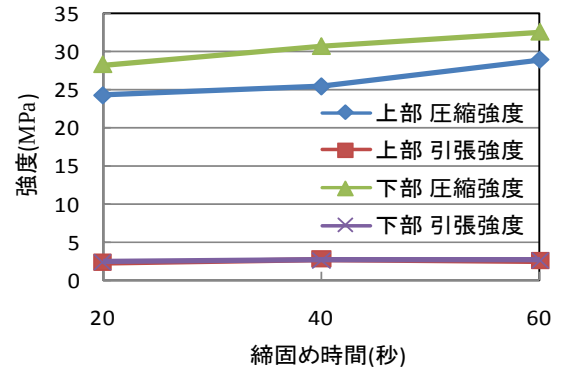
図-3 合板型枠スランプ 8cm による場合
