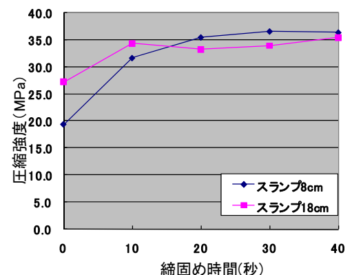
図-1 締固め時間の変化による圧縮強度
