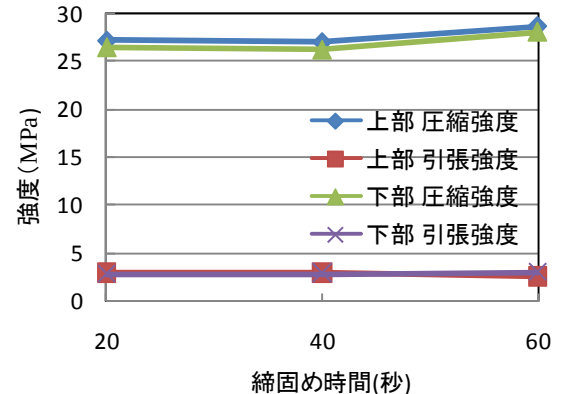
図-6 ラス型枠スランプ 18cm による場合
