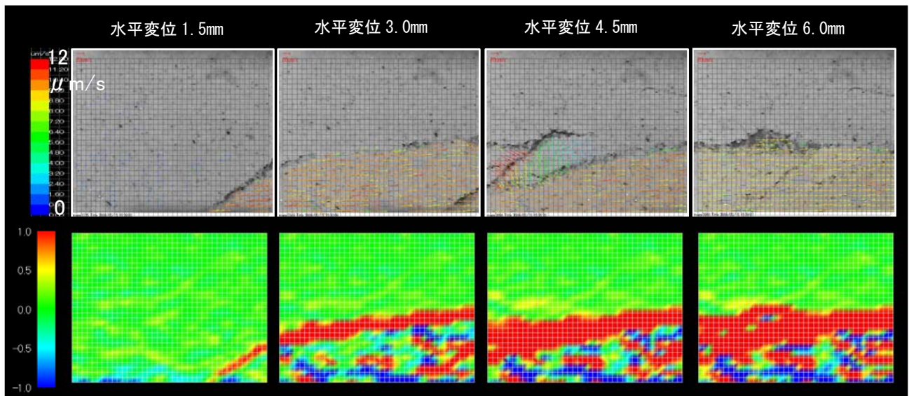
図3 正規圧密供試体のせん断過程におけるせん断帯の観察： (a)速度ベクトル(上図)，(b)せん断ひずみ(下図)
