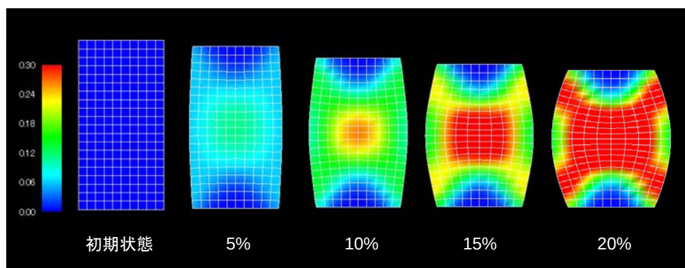
図 2 境界非排水条件下の平面ひずみ圧縮中のせん断ひずみ分布
