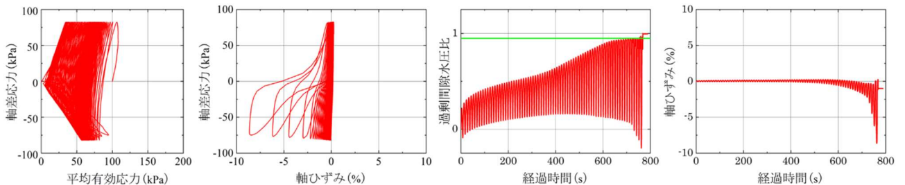
図5 改良供試体 (改良3: 相対密度40%, 繰返し応力比0.400)
