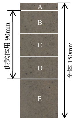
図2 供試体の各区間名
