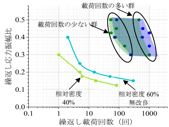
図3 液状化強度曲線
