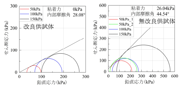
図7 CUB試験結果 (相対密度60%)
