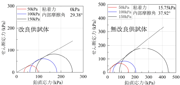
図6 CUB試験結果 (相対密度40%)
