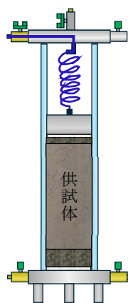
図1 改良供試体の模式図
