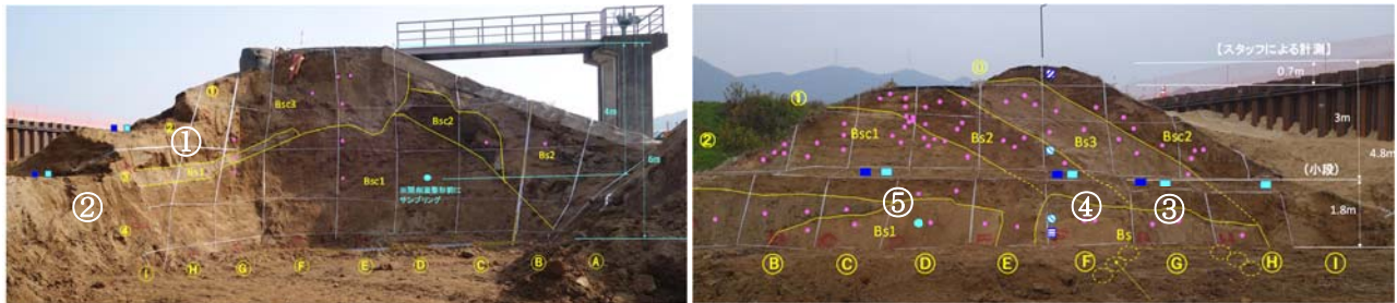
図2 右岸 0.6k の破堤箇所における開削調査時の現場透水試験の実施箇所（左：上流断面，右：下流断面）
