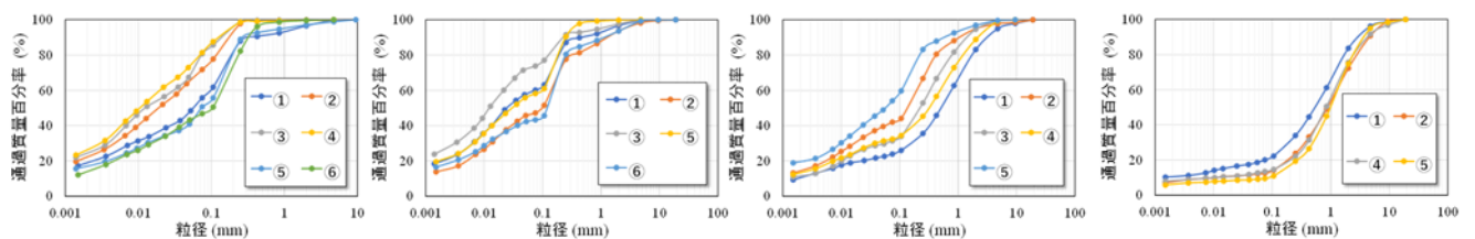
図4 左岸 6.4k 地点での現場と室内の粒径加積曲線 (左：現場透水試験近傍，右：室内透水試験から)
