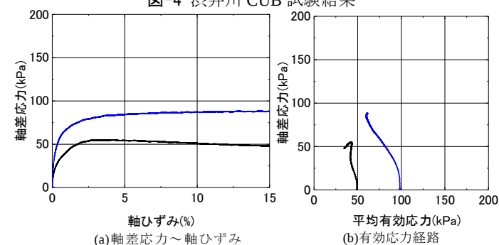
図-5 ニッ森川 CUB 試験結果
