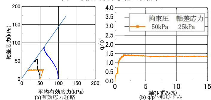
図-7 ニッ森川吸水軟化試験結果
