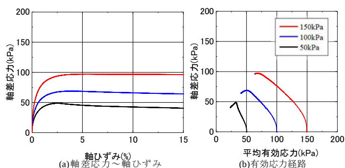
図-4 渋井川 CUB 試験結果
