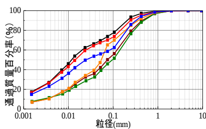
図-1 渋井川試料の粒度分布
