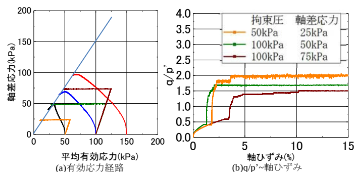
図-6 渋井川吸水軟化試験結果
