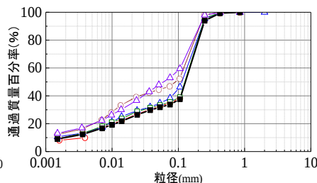
図-2 ニッ森川試料の粒度分布
