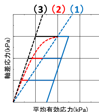
図 3 吸水軟化試験の有効応力経路
