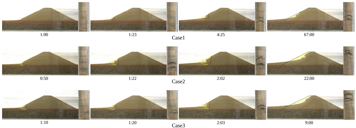
図 2 堤体模型の変状および実験終了時の様子（図中の数字は経過時間 m:s）
