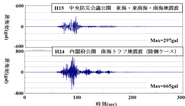
図 3 解析に用いた入力地震動
