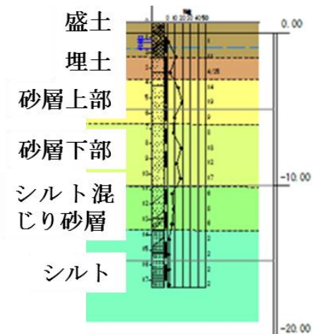
図 1 解析に用いた地盤モデル
