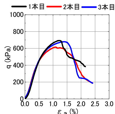
(a) 固化供試体 養生7日
