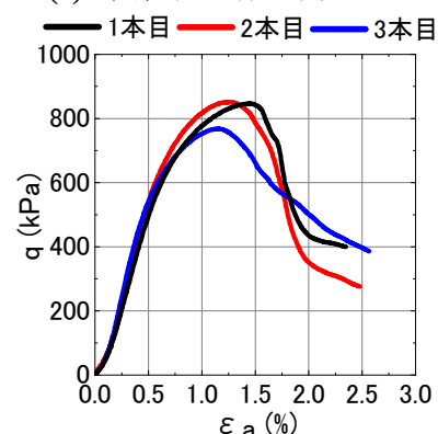
(b) 固化供試体 養生14日
