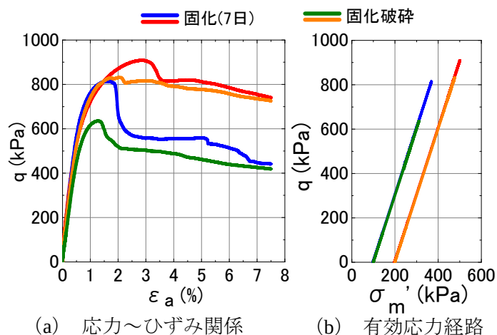
図 2 三軸 CD 試験結果
