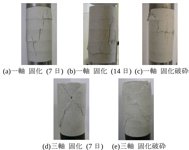
写真 1 試験後の供試体の様子
