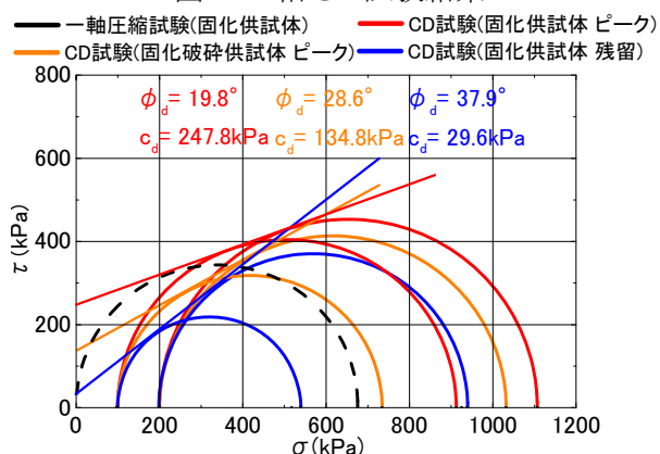
図 3 試験方法別のモールの応力円
