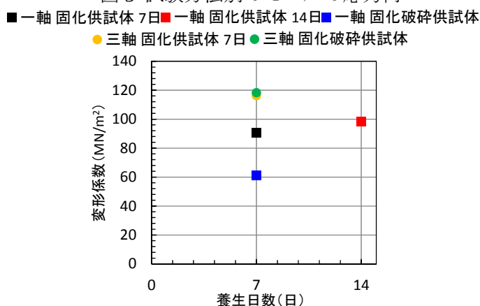
図 4 養生日数と変形係数の関係
