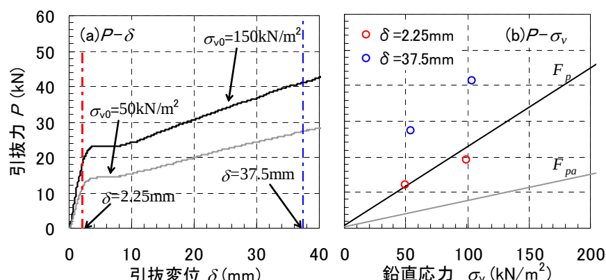
図-2 支圧単体補強材の引抜結果
