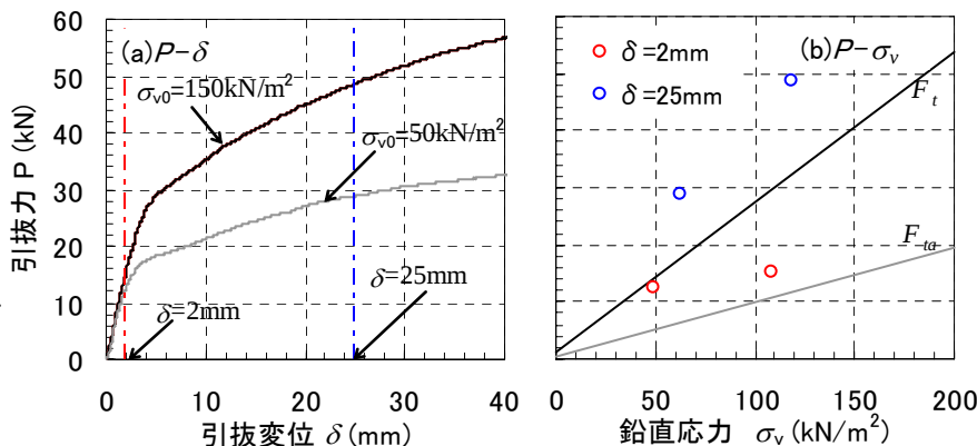
図-4 併用補強材の引抜結果
