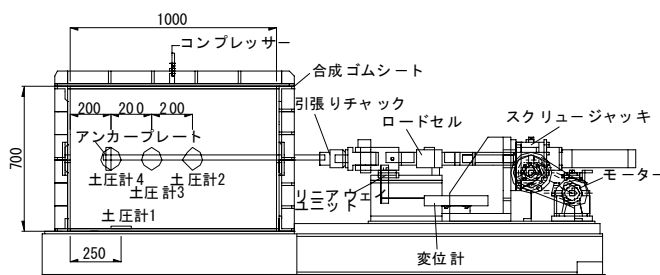
図－1 小型土中引抜試験機の断面図
