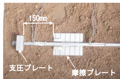
写真－1 併用補強材
