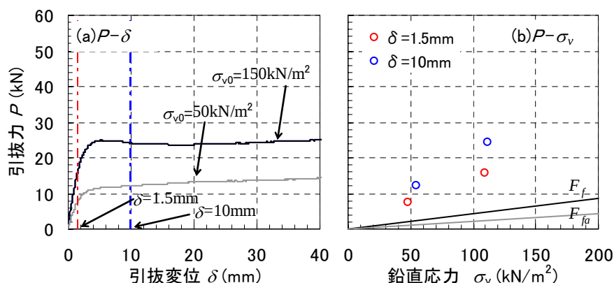
図-3 摩擦単体補強材の引抜結果
