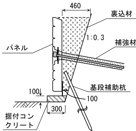
図-3 基本段の施工断面図
