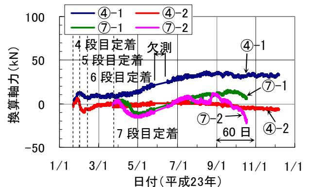
図-5 補強材軸力の推移(4段目,7段目)
