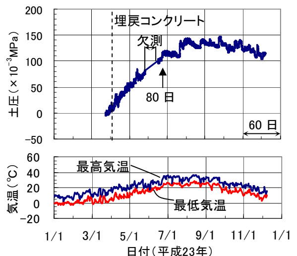
図-6 壁面真下の鉛直土圧と気温変化
