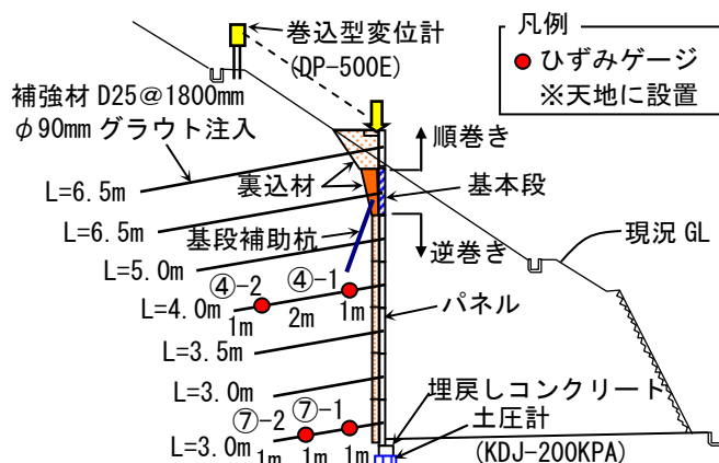
図-1 実大実験施工断面図と動態観測位置図
