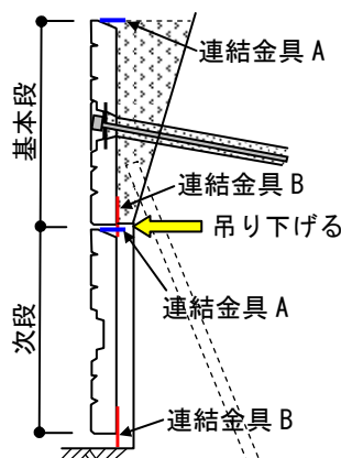
図-4 基本段と次段の連結
