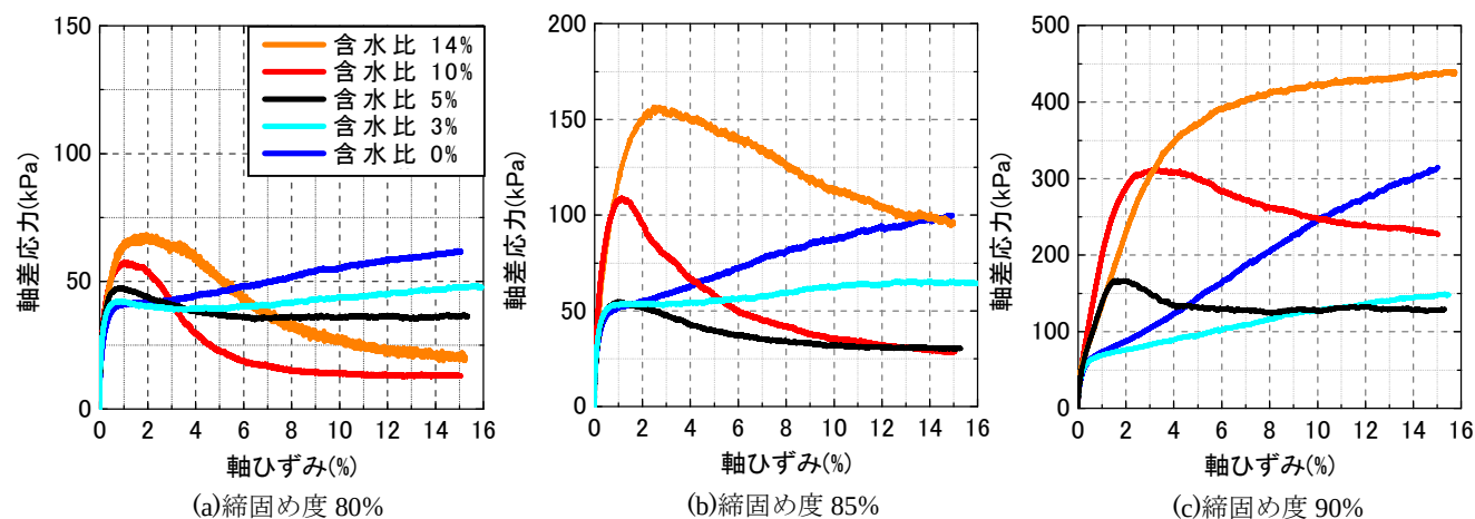
図 2 応力～ひずみ関係
