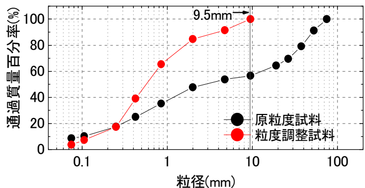
図1 実験試料の粒度分布
