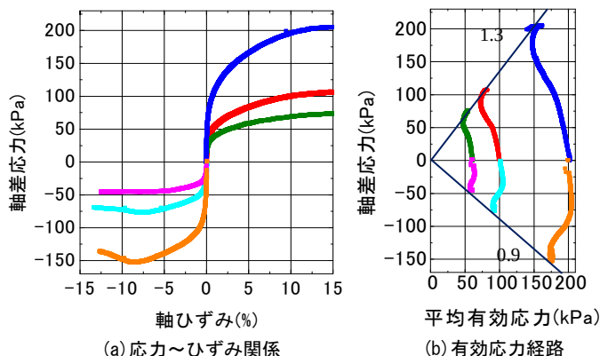
図4 練り返し粘土を用いた三軸試験結果
