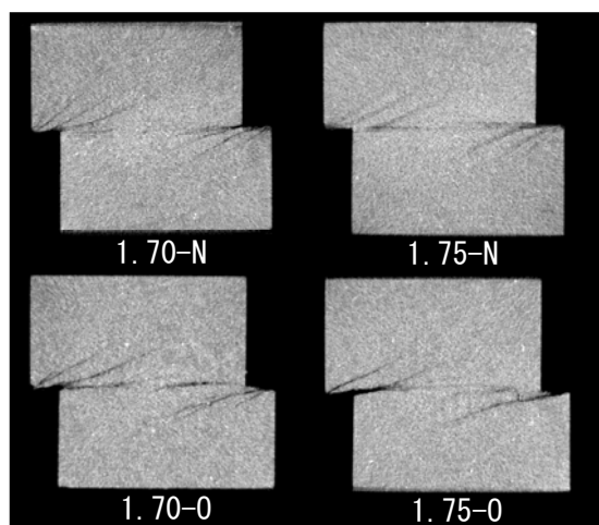
(a) 密度を変化させた供試体
