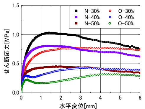
(a) せん断応力～変位関係
